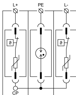
Schemat okablowania wewnętrznego
