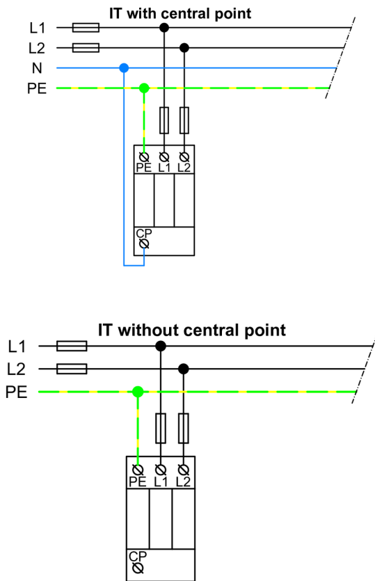
Schemat okablowania aplikacji (instalacja)
